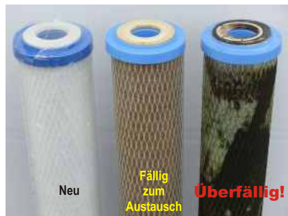
Abb.2: Aktivkohleblock-Filter 10µ.
